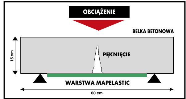
Rys. 1 Wykonanie izolacji Mapelastic na belce betonowej narażonej na działanie obciążeń zginających.
