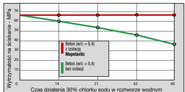
Rys. 4 Wpływ izolacji Mapelastic na ograniczenie spadku wytrzymałości betonu spowodowanego działaniem soli odładzających, zawierających chlorek wapnia.
